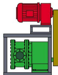
3 – Toppmonterad remdrift
