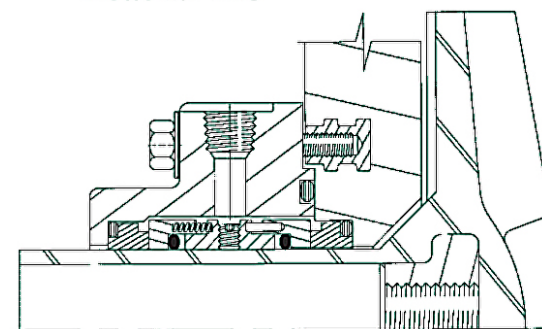
FLOWERVE RXO
